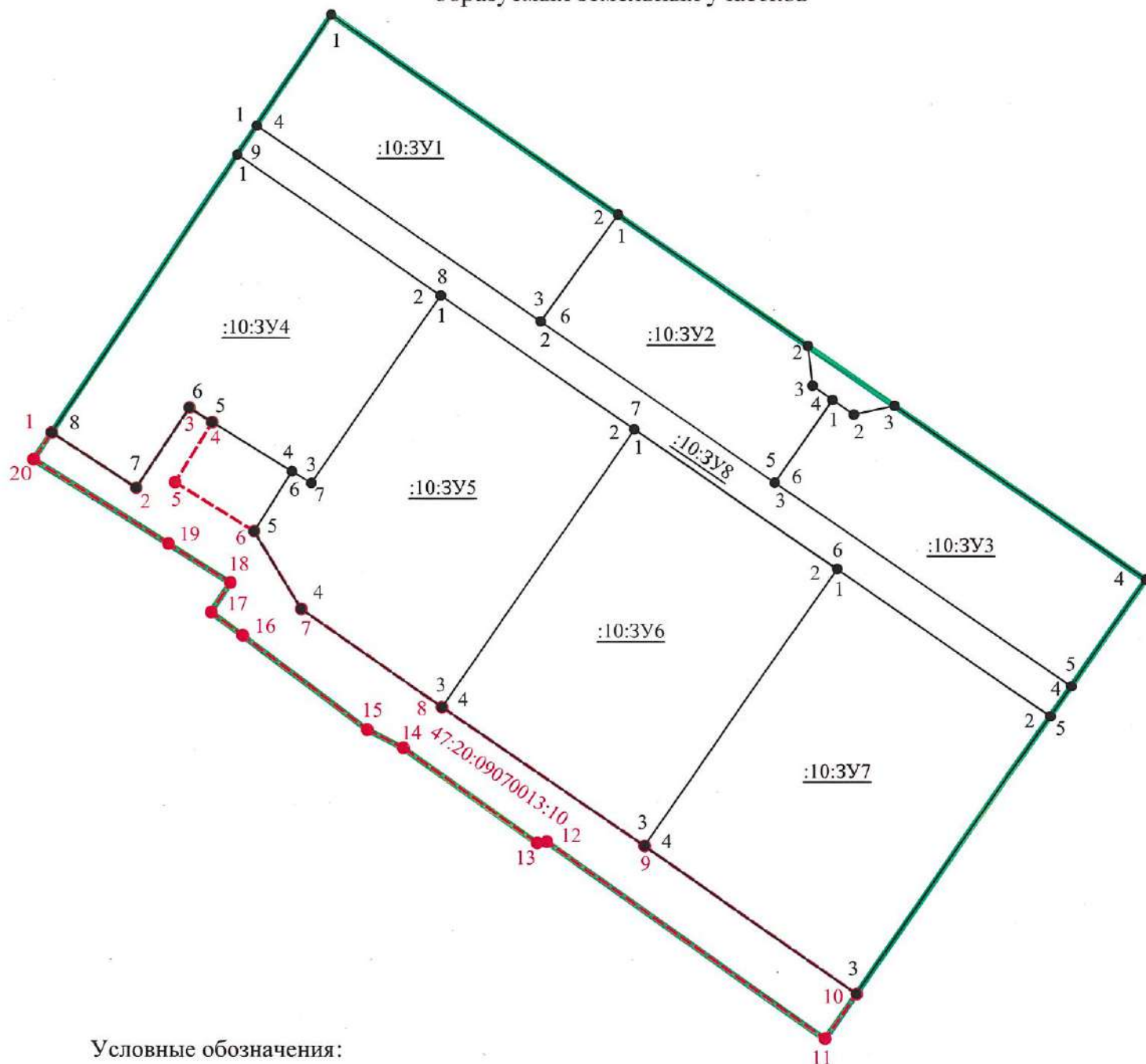
Чертеж межевания территории, отображающий границы изменяемых и образуемых земельных участков
