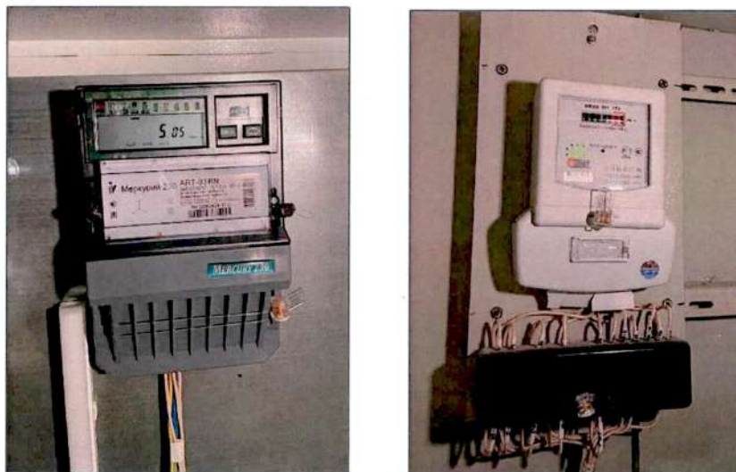
Рисунок 5.3.3 – Приборы учета электрической энергии
